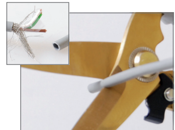
Odizolování vodičů
