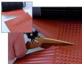
Stříhání hliníku
